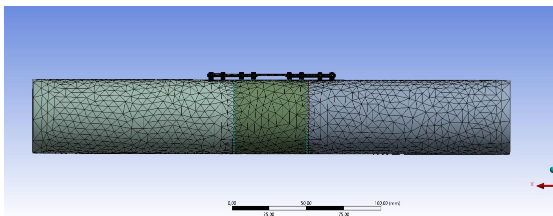
Rys. 6. Model po dokonaniu podziału na elementy skończone.
