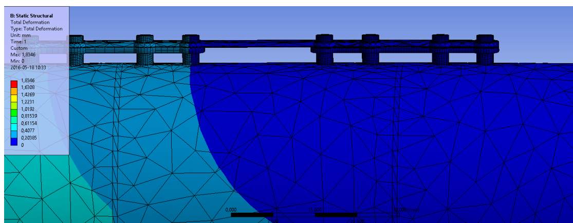
Rys. 10. Zobrazowanie przemieszczeń występujących na stabilizatorze.
