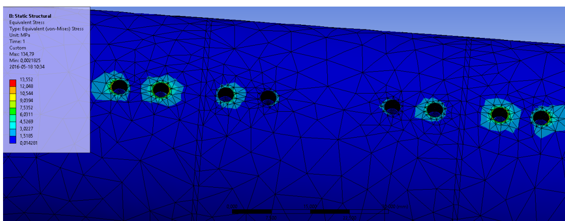
Rys. 11. Zobrazowanie naprężeń zredukowanych von Misesa występujących w miejscach wkręcenia stabilizatora w kość.
