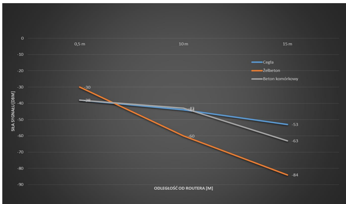
Rysunek. 10. Wykres przedstawiający porównanie siły sygnału sieci bezprzewodowej wraz z zastosowanym materiałem na budowę ścian budynku
