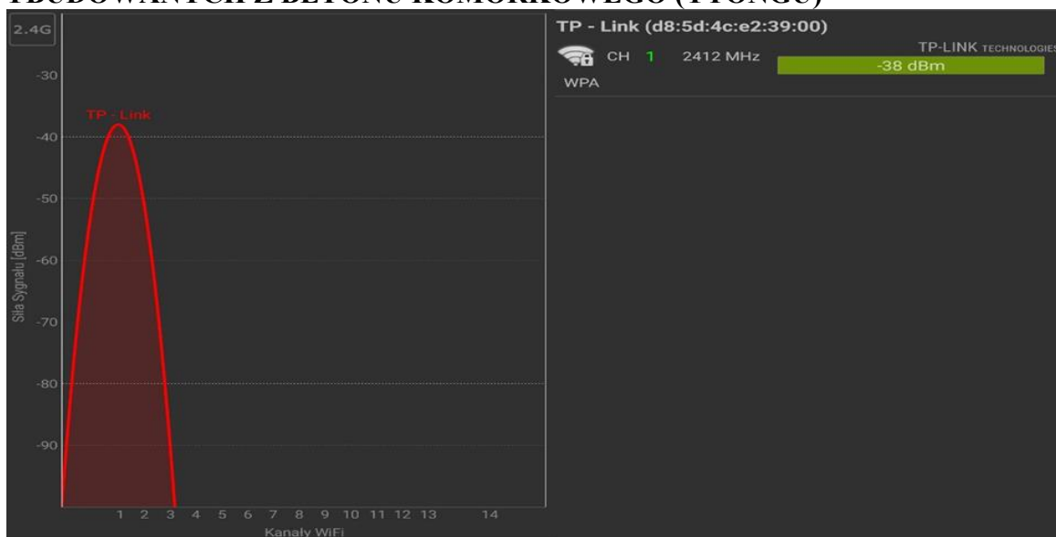
Rysunek. 7. Wykres siły sygnału sieci bezprzewodowej WiFi w odległości 0,5 metra od routera dla ścian wybudowanych z betonu komórkowego.
