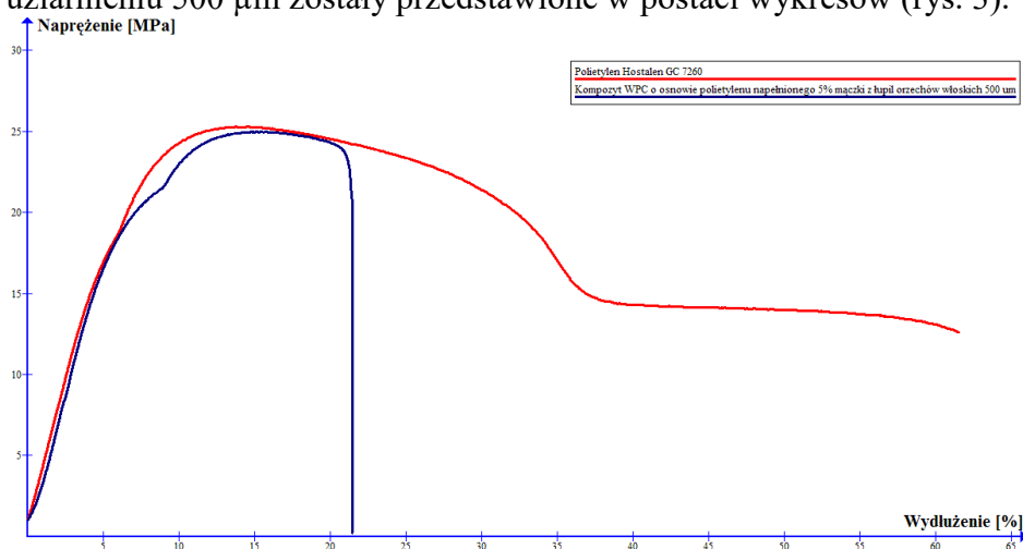
Rys. 3. Wyniki statycznej próby rozciągania czystego polietylenu Hostalen GC 7260 i kompozytu WPC o osnowie polietylenu napełnionego 5% mączki z łupin orzechów włoskich o wielkości ziarna 500 \mu m.
