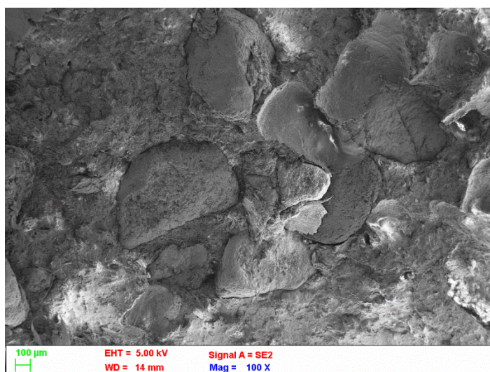
Rys. 4. Zdjęcie przełomu kompozytu WPC o osnowie polietylenu napełnionego 10% mączki z łupin orzechów włoskich o uziarnieniu 500 \mu\text{m} (SEM, Zeiss Supra 55), powiększenie.
