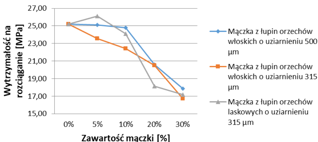
Rys. 5. Zestawienie maksymalnych wytrzymałości na rozciąganie kompozytu WPC
