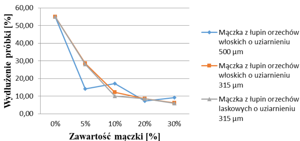
Rys. 8. Zestawienie maksymalnego wydłużenia próbek podczas statycznego rozciągania kompozytu WPC
