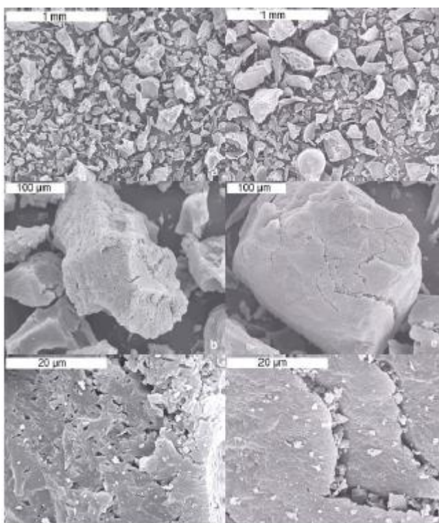
Rys. 2. Zdjęcia SEM ziaren węgla aktywnych[5]. Fig. 2. SEM image of activated carbon grains[5].
