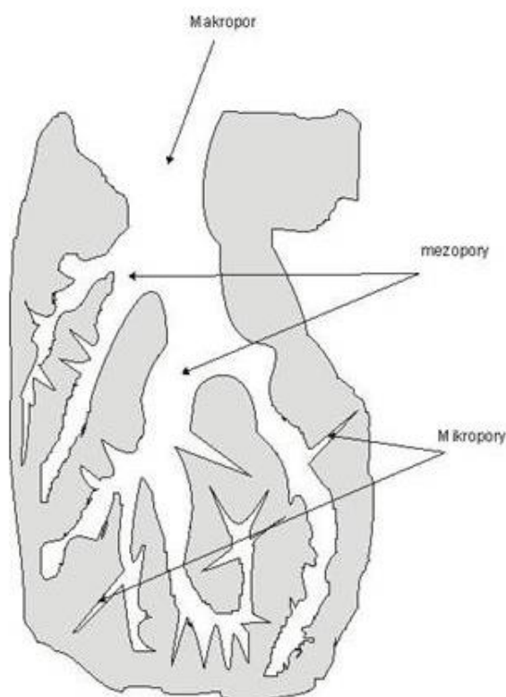
Rys. 4. Rozkład porów w węglu aktywnym po procesach karbonizacji i aktywacji[11]. Fig. 4. Pore distribution in activated carbon after carbonization and activation processes[11].
