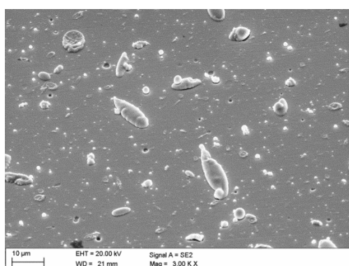
Rys. 5. Topografia powłoki \text{Al}(\text{TiN-ZrN})_{x5}
