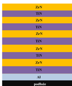
Rys. 1. Schemat powłoki wielowarstwowej Al(TiN-ZrN) x5
