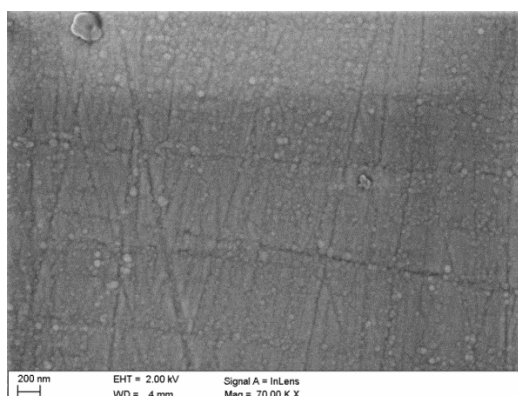
Rys. 7. Topografia powłoki \text{Al}_2\text{O}_3
