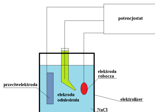
Rys. 2. Schemat stanowiska do wykonywania badań odporności na korozję elektrochemiczną Fig. 2. Equipment used for corrosion test
