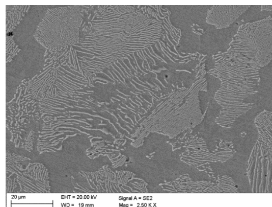
Rys. 4. Struktura podłoża na mikroskopie skaningowym
