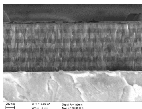
Rys. 6. Wielowarstwowa struktura powłoki PVD
