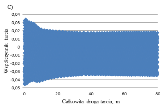
Rys. 3. Współczynnik tarcia dla: C) – próbki starzonej płynem do płukania jamy ustnej Listerine
