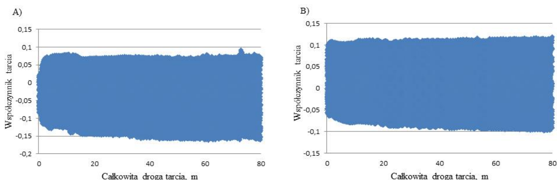
Rys. 2. Współczynnik tarcia dla: A) – próbki starzonej wodą dejonizowaną, B) – próbki starzonej alkoholem etylowym o stężeniu 75%
